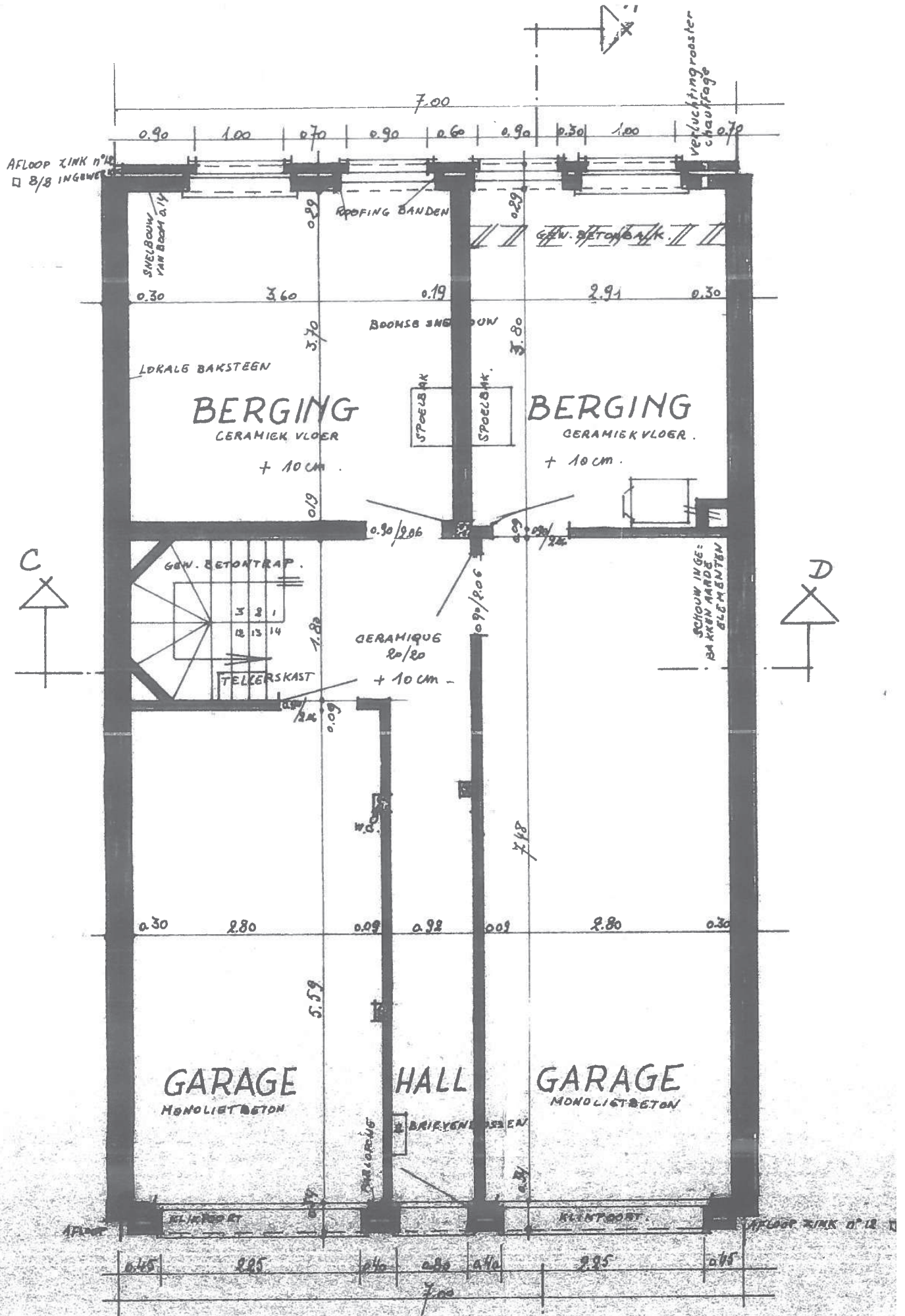
GRONDPLAN
